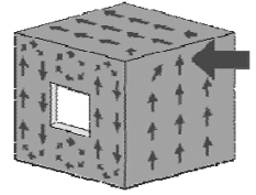
モノコック工法のイメージ
